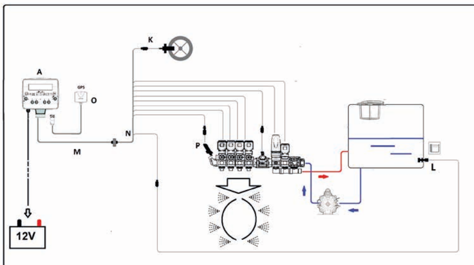
Example: Orchard 4 sections connection diagram Ejemplo: esquema de conexión Orchard de 4 secciones Exemplo: esquema de ligação Orchard de 4 secções
